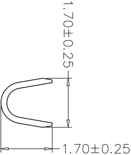
SEC:B-B
